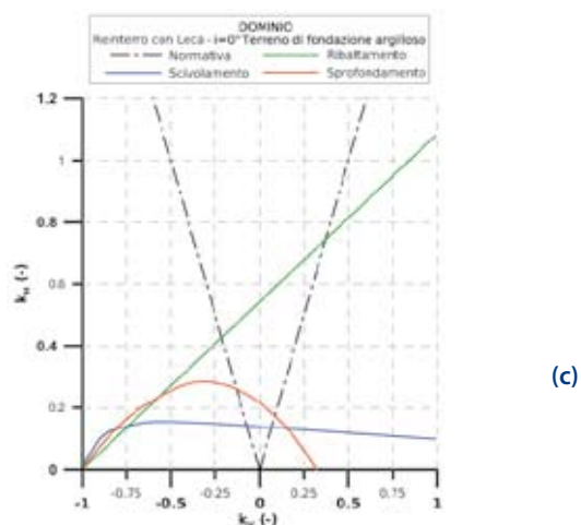
Figura 10 Dominio ( i=0^\circ ) in presenza di terreno di fondazione di proprietà scendenti e (a) reinterro in materiale non alleggerito; (c) reinterro con Leca e (e) reinterro con Leca e muro in calcestruzzo alleggerito. (b; d-, f) confronto con le accelerazioni di Normativa.
