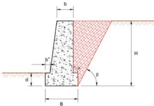
Figura 2 Schema geometrico di un muro di sostegno a gravità.
