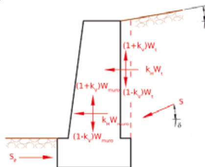
Figura 5 Schema pseudostatico del muro; pendio inclinato.
