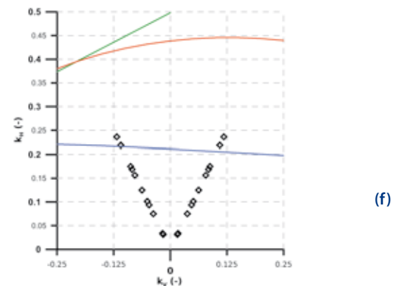
Figura 10 Dominio ( i=0^\circ ) in presenza di terreno di fondazione di proprietà scendenti e (a) reinterro in materiale non alleggerito; (c) reinterro con Leca e (e) reinterro con Leca e muro in calcestruzzo alleggerito. (b; d-, f) confronto con le accelerazioni di Normativa.
