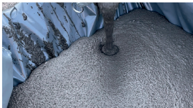
Iniezioni all'intradosso della calotta in galleria sull'Autostrada A30 a Salerno. Anno 2021. • Leca Inject • ReoLeca.
