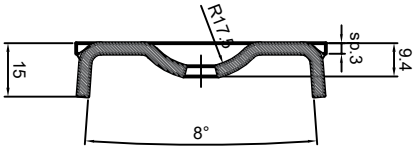
A-A (1 : 1)
